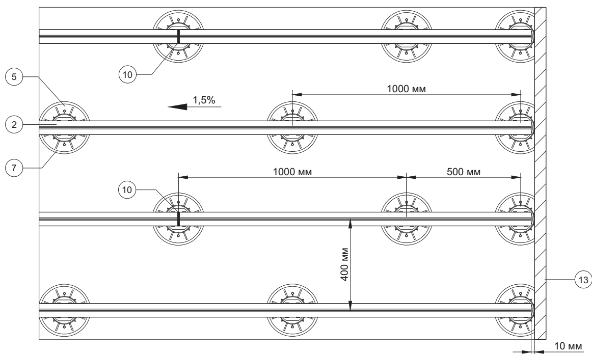
Вид сверху
