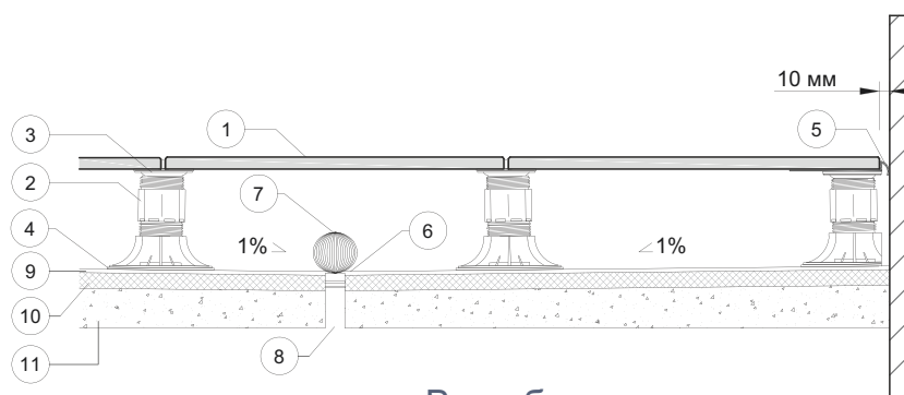
Вид сбоку
