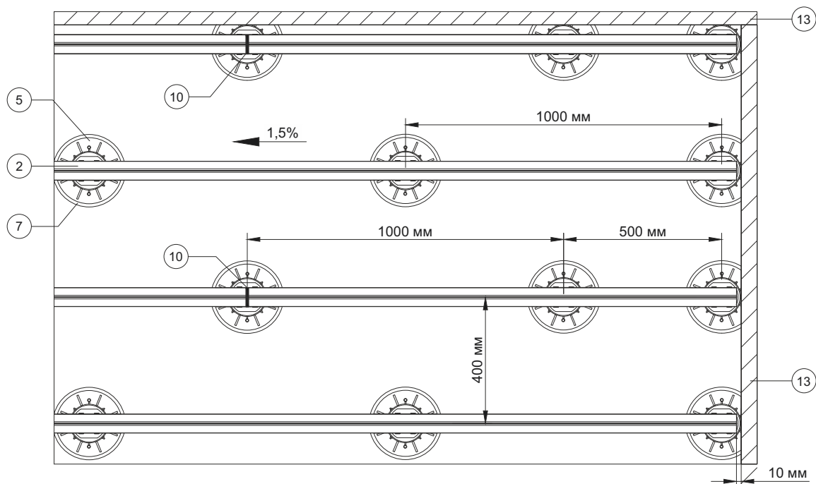
Вид сверху
