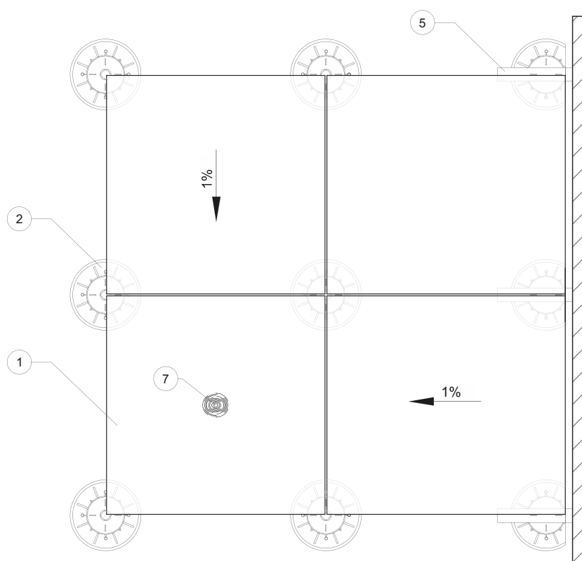
Вид сверху
