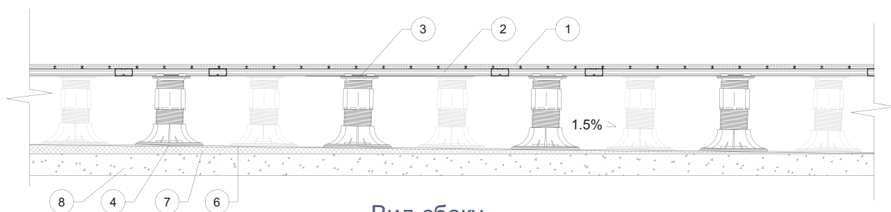
Вид сбоку
